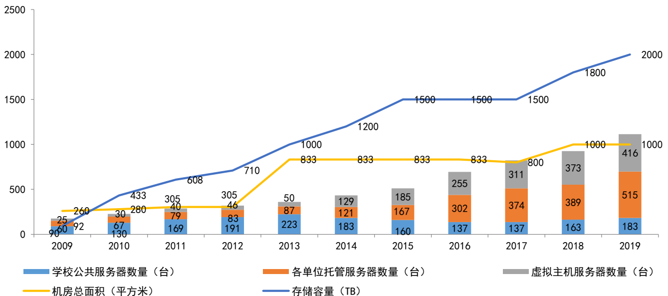
2009-2019年IDC机房基础设施建设情况
